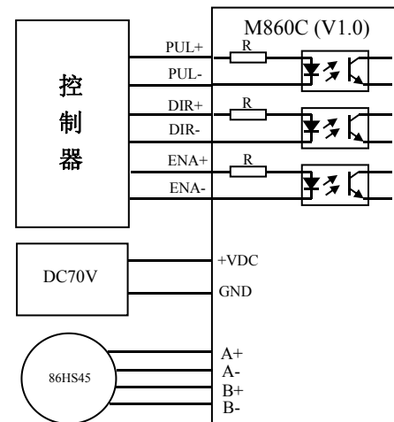
图 6 M860C (V1.0)配 86 电机典型接法
